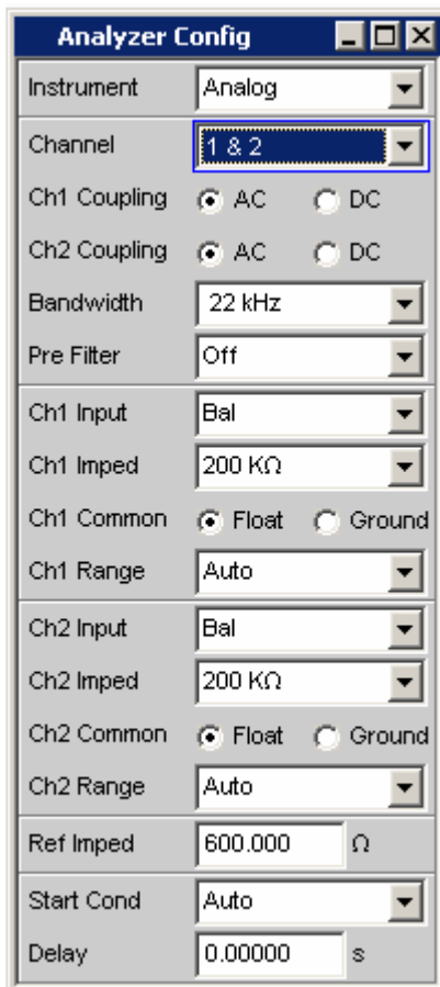
Bild 4-11 Analyzer-Config-Panel
