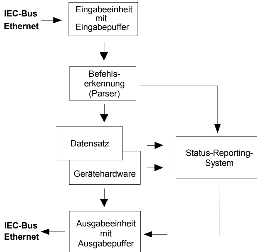
Bild 5-2 Gerätemodell bei Fernsteuerung über IEC-Bus oder TCP/IP-Netzwerk
