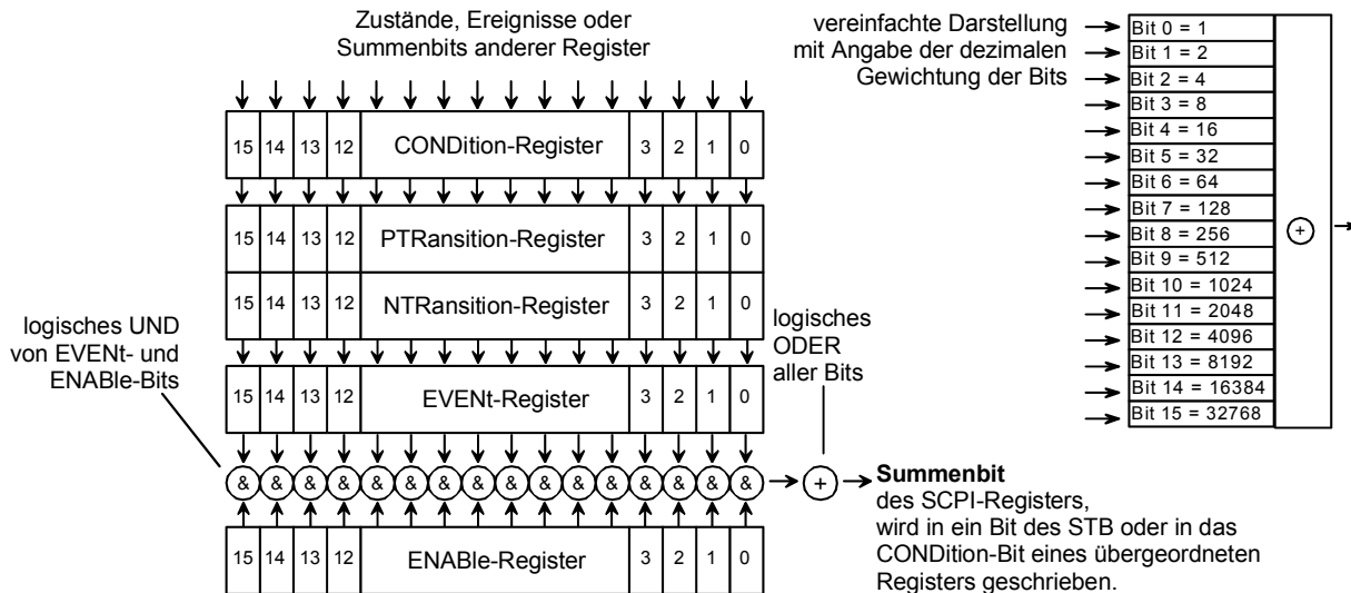
Bild 5-3 Standard SCPI-Statusregister
