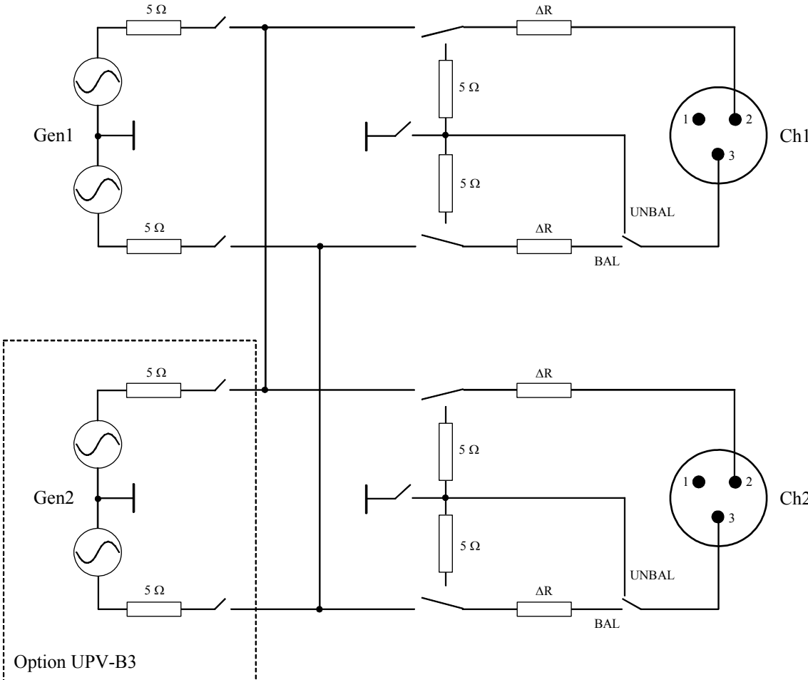
Bild 4-9 Beschaltung der Ausgänge bei DIM Beide Generator-Ausgänge werden von der Option R&S UPV-B3 (Second Generator) gespeist.
