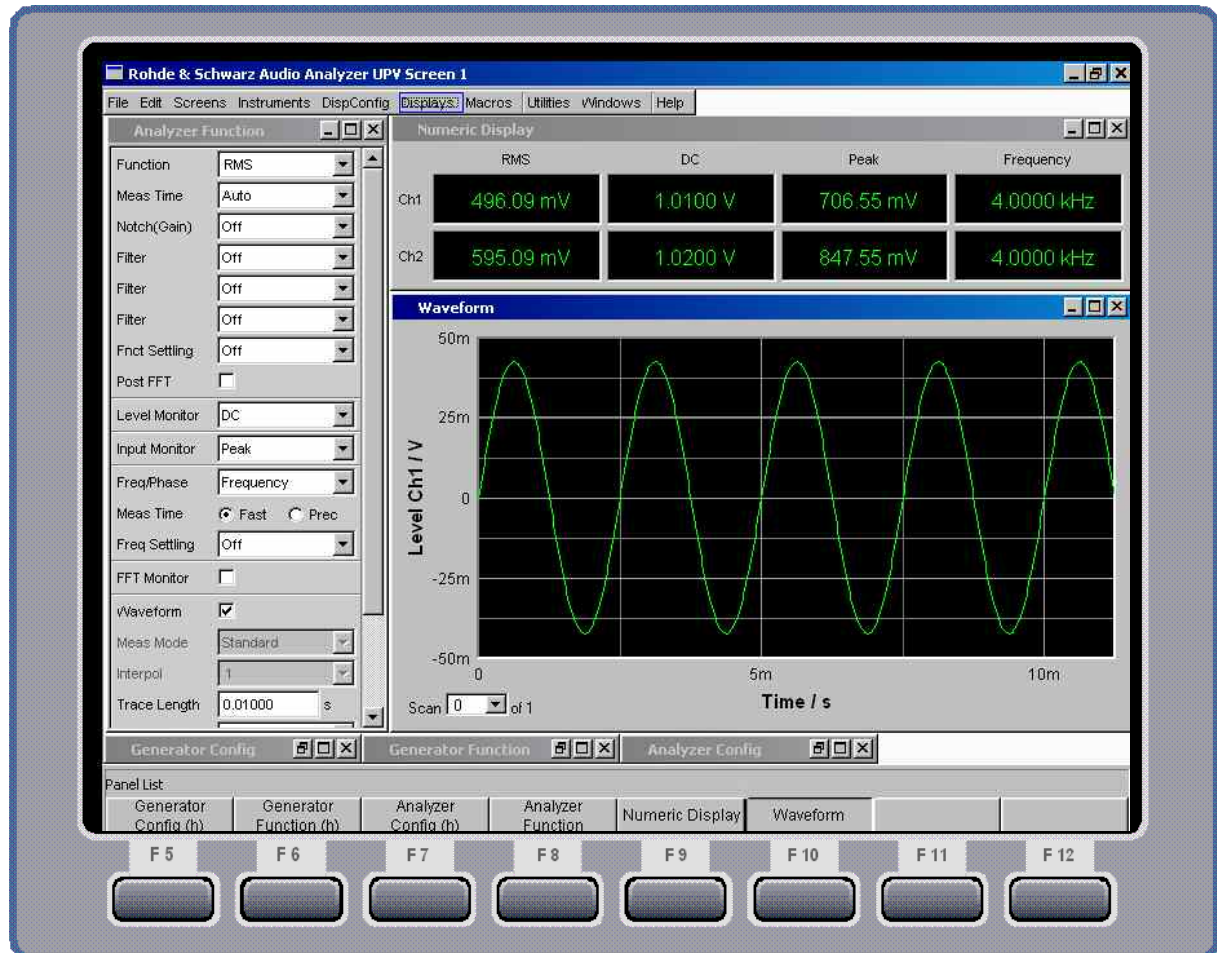
Bild 1-2 Bildschirm
