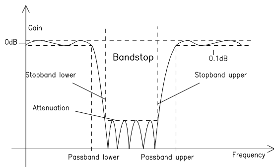
Bild 4-29 Band Stop Frequenzgang mit Kennzeichnung der Filterparameter
