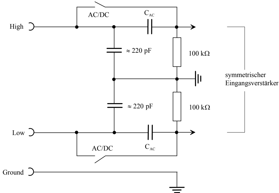
Bild 4-16 Symmetrischer Analyzer-Eingang
