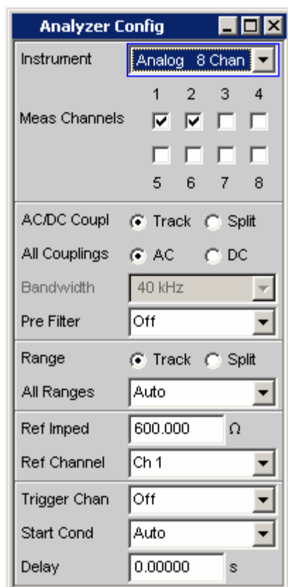
Bild 4-15 Multi-Kanal Analyzer-Config-Panel
