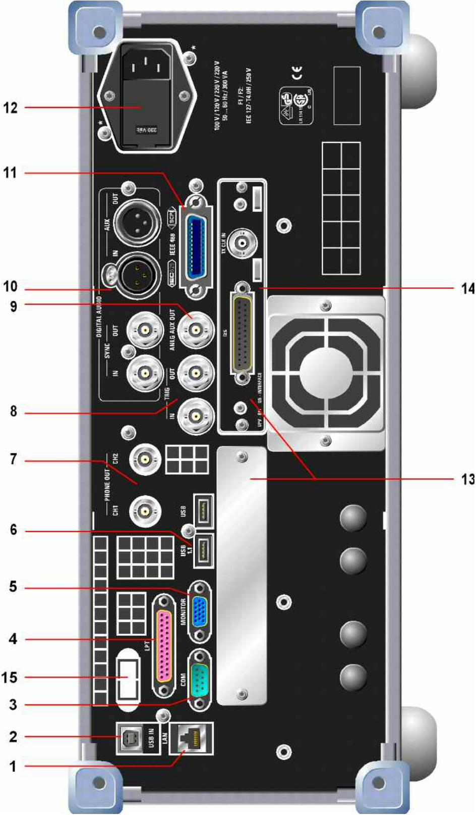
Bild 1-3 Rückansicht
